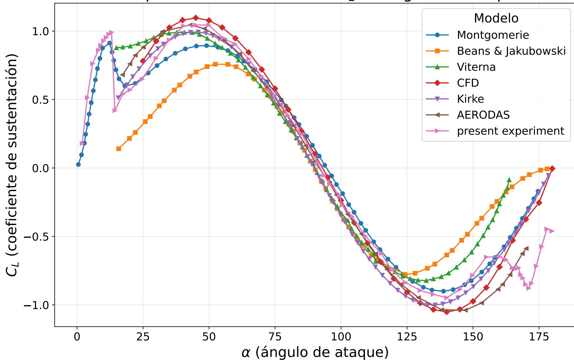
Comparación de modelos de C_L vs Ángulo de ataque
